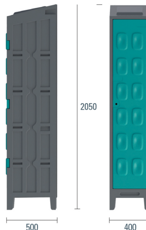
Casier vestiaire qualité alimentaire avec une étagère tringle + cloison réglable 3 points
